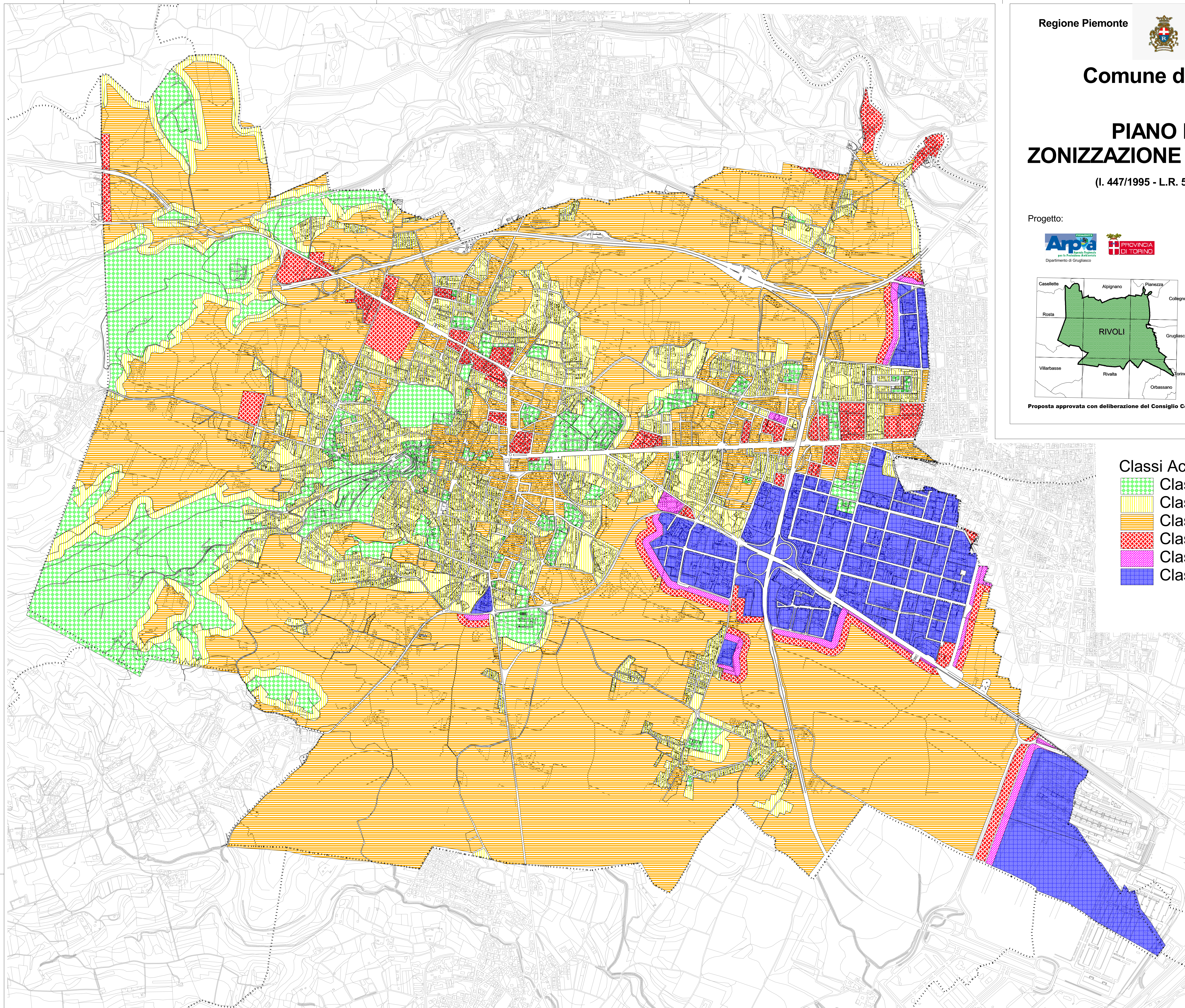
Tavola 1: Planimetria generale
